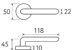
D1 Дверная ручка на круглом основании 5 ЛЕТ ГАРАНТИИ Латунь Алюминий ЦАМ
