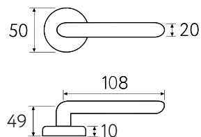
D1 Дверная ручка на круглом основании 5 ЛЕТ ГАРАНТИИ Латунь Алюминий ЦАМ
