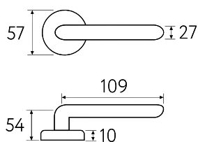
D8 Дверная ручка на круглом основании 5 ЛЕТ ГАРАНТИИ
