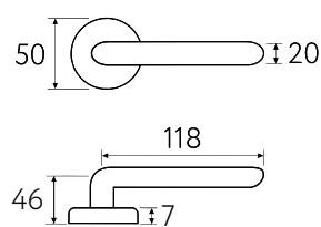
7.7 Дверная ручка на круглом основании 5 ЛЕТ ГАРАНТИИ Латунь Алюминий ЦАМ
