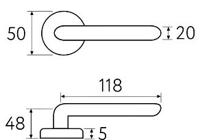
7FS Дверная ручка на круглом основании 5 ЛЕТ ГАРАНТИИ Латунь Алюминий ЦАМ
