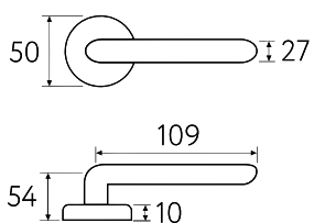
D1 Дверная ручка на круглом основании 5 ЛЕТ ГАРАНТИИ
